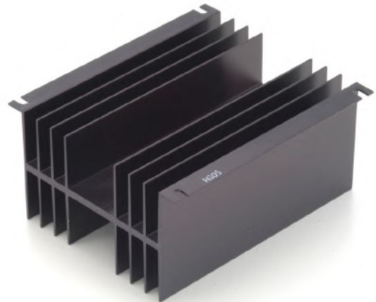
HS05 0.85°C/W
